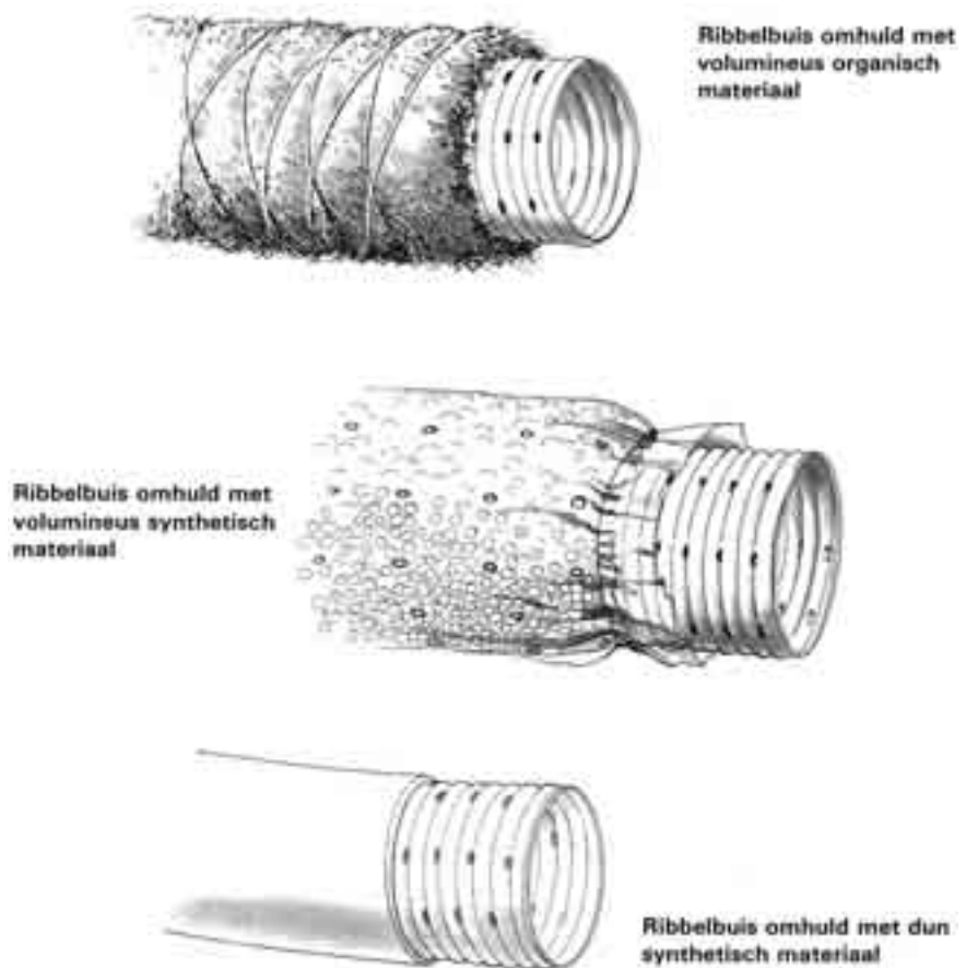
Fig. 6.1 Omhuilingsmateriaal zorgt ervoor dat fijne gronddeeltjes niet in de drain komen.
