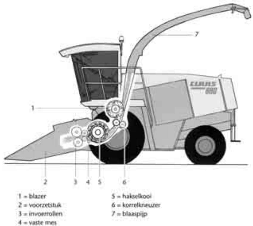
Fig. 12.2 Onderdelen van een zelfrijdende hakselaar
