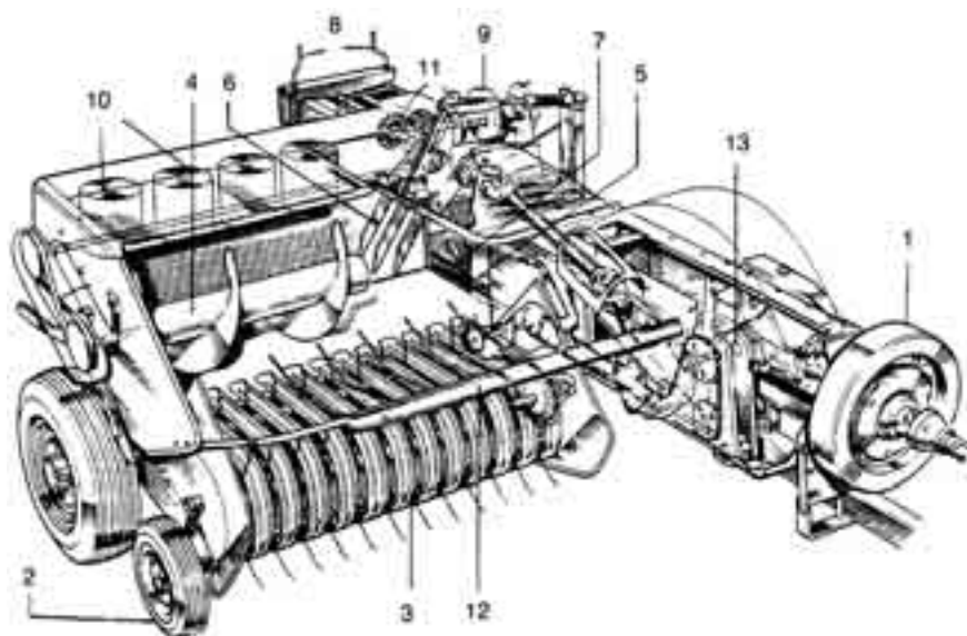
Fig. 11.2 De onderdelen van een opdraapers
