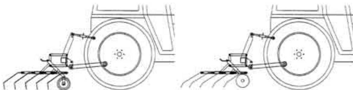
Fig. 4.7 De tanden kunnen stekend (links) of slepend (rechts) ingesteld worden.
