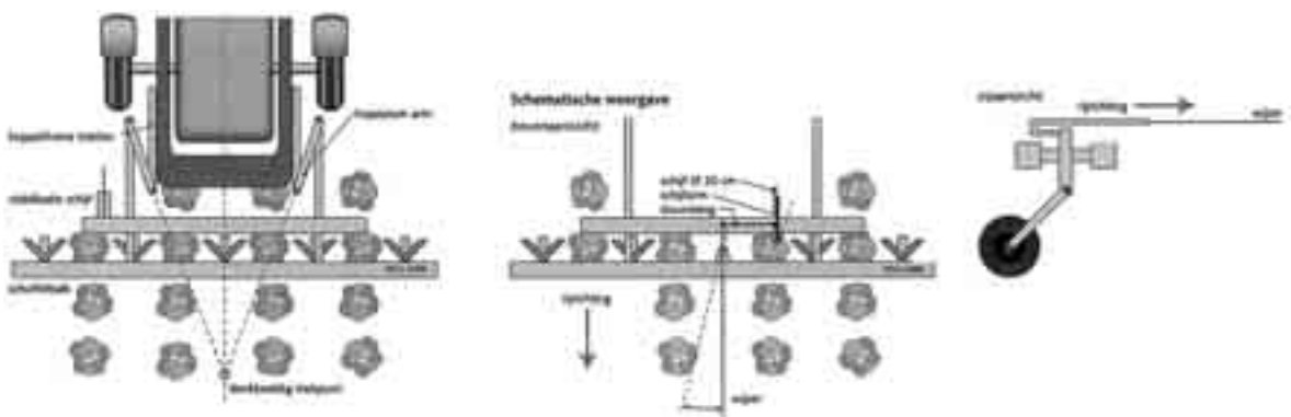
Fig. 4.21 Bij een frontschoffel met wijzersysteem kan de bestuurder snel en eenvoudig vooraf corrigeren.
